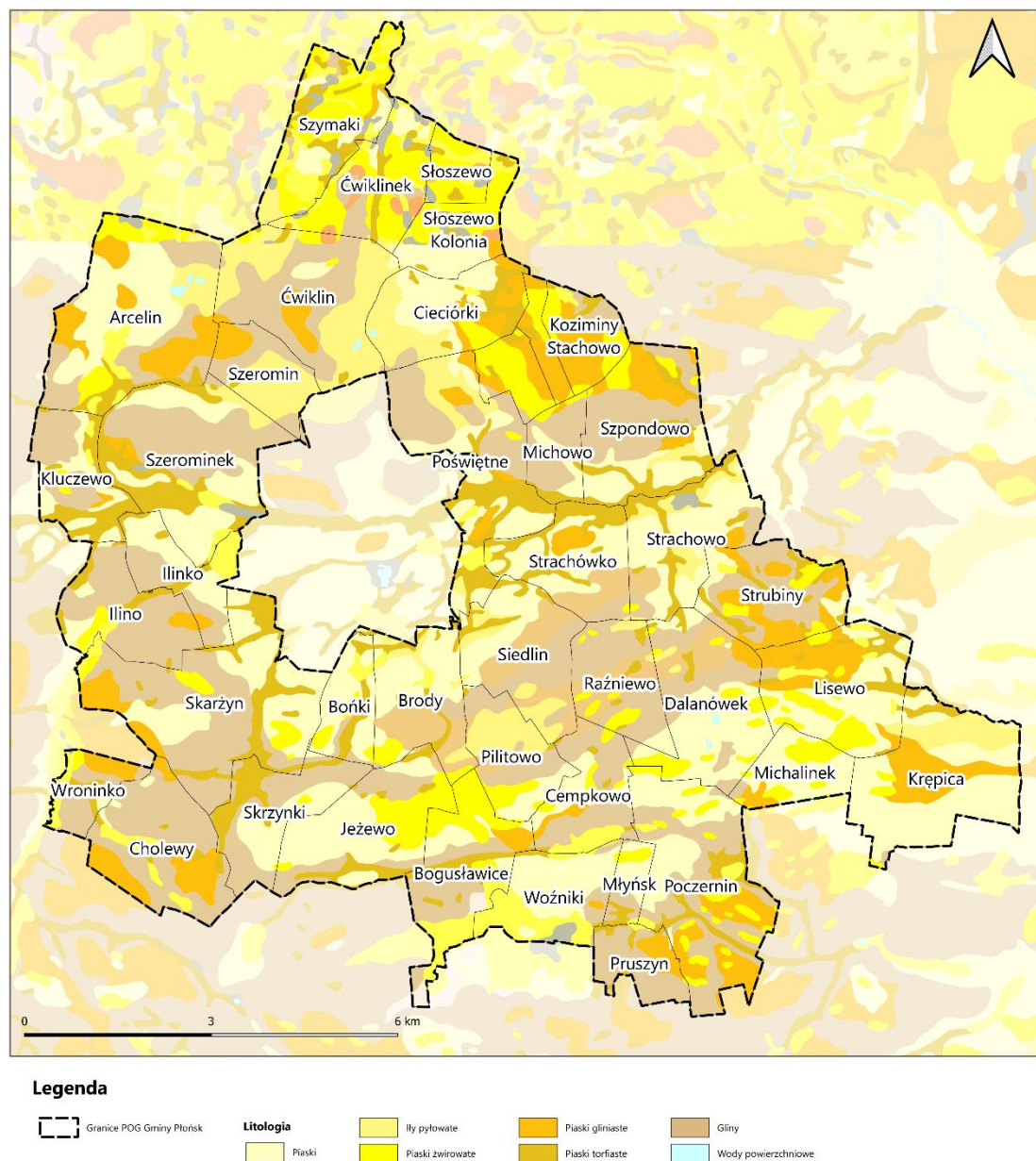
Ryc. 13 Mapa litogenetyczna
